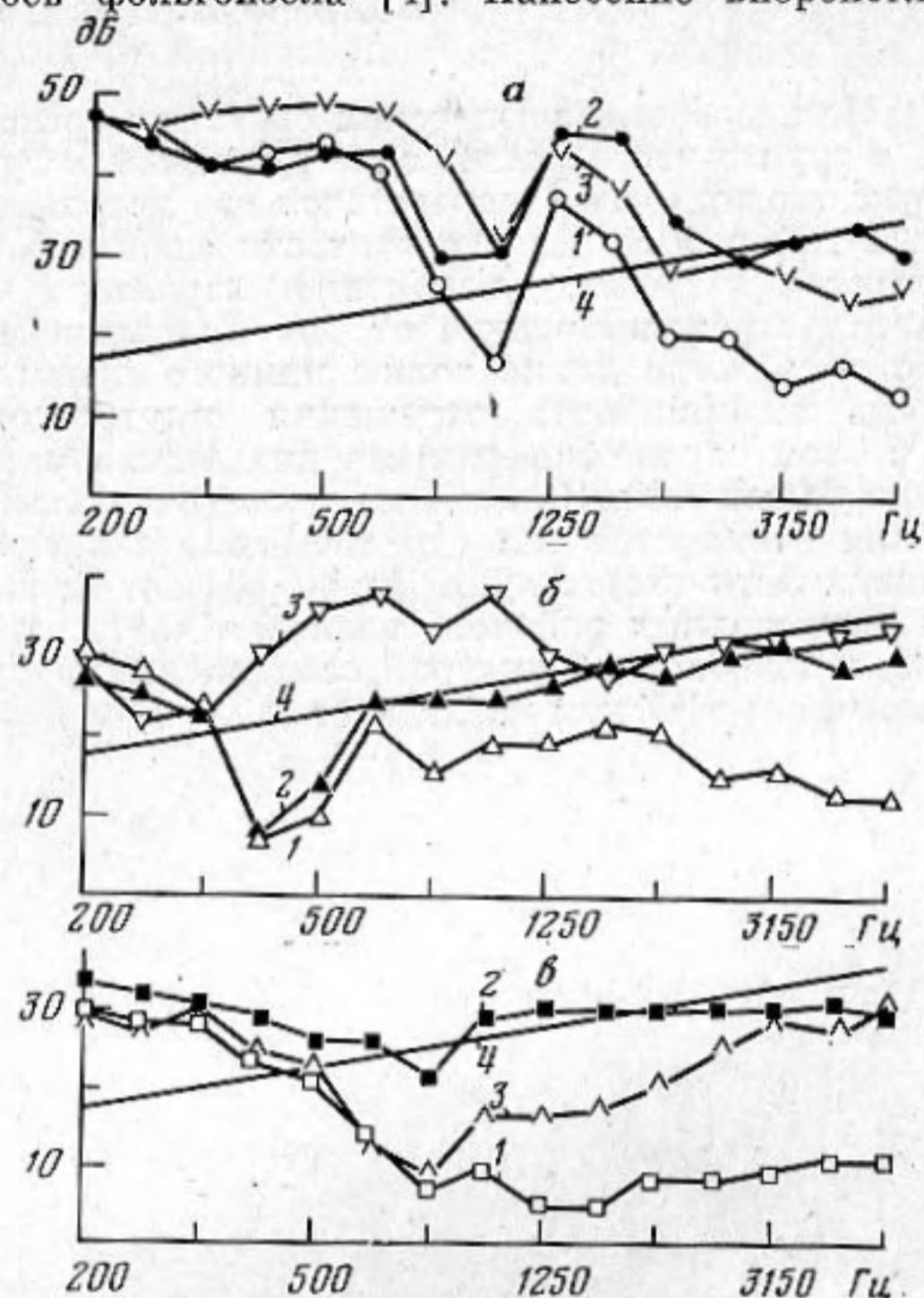
Звукоизоляция оболочек различной формы: а — сферической, б — цилиндрической, в — прямоугольной, 1 — звукоизоляция полой оболочки, 2 — звукоизоляция оболочки со звукопоглощающим покрытием, 3 — звукоизоляция оболочки с вибропоглощающим покрытием, 4 — звукоизоляция пластины «по закону массы»
