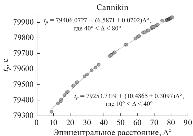
Рис. 4. Годограф для фаз iP/eP испытания Cannikin.
