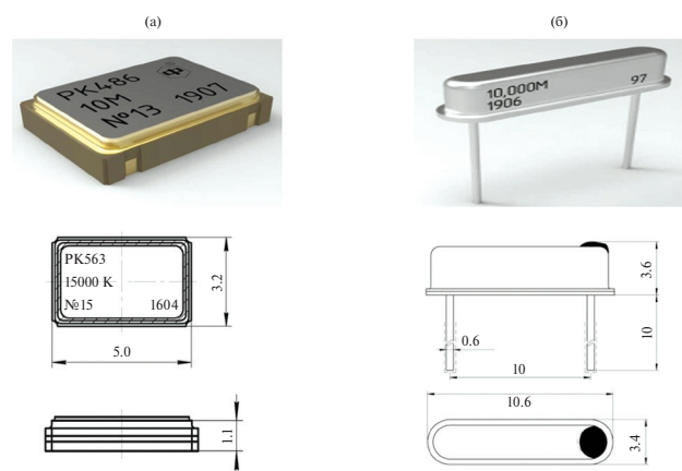
Рис. 1. Общий вид и габаритные размеры резонаторов (а) — РК563 (тип 1) в корпусе поверхностного монтажа и (б) — РК319 (тип 2) в корпусе четвертьволнового резонатора.
