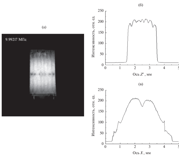
Рис. 4. (а) — Топограмма и (б), (в) — графики распределения по двум направлениям амплитуды деформаций пьезоэлемента на резонансной частоте 9.99217 МГц, соответствующей 1-ой гармонике.
