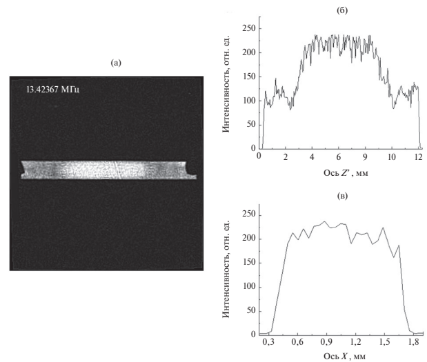
Рис. 10. (а) — Топограмма и (б), (в) — графики распределения по двум направлениям деформаций пьезоэлемента на резонансной частоте 13.42367 МГц, соответствующей ангармоническому колебанию.
