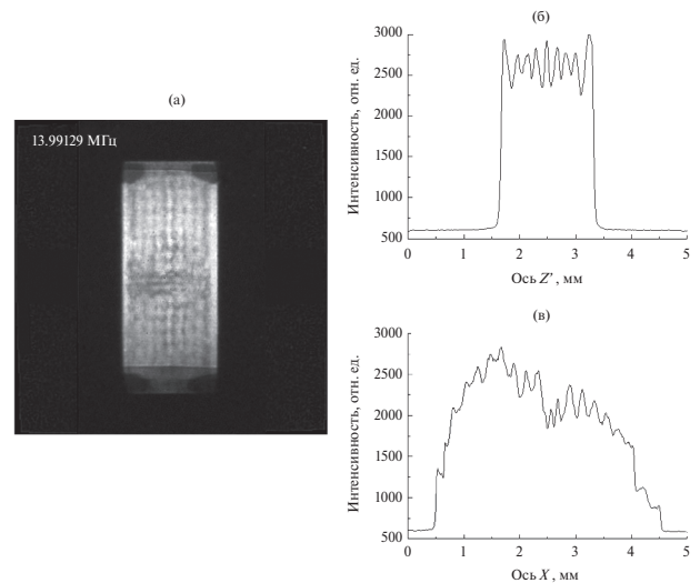
Рис. 7. (а) — Топограмма и (б), (в) — графики распределения по двум направлениям амплитуды деформаций пьезоэлемента на резонансной частоте 13.99129 МГц, соответствующей 1-ой гармонике.
