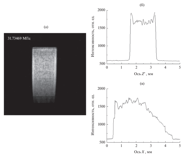
Рис. 5. (а) — Топограмма и (б), (в) — графики распределения по двум направлениям амплитуды деформаций пьезоэлемента резонатора 1-го типа на резонансной частоте 31.73469 МГц, соответствующей 3-ей гармонике.
