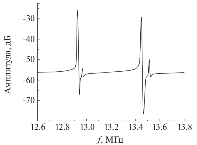
Рис. 8. Амплитудно-частотная характеристика резонатора 2-го типа.
