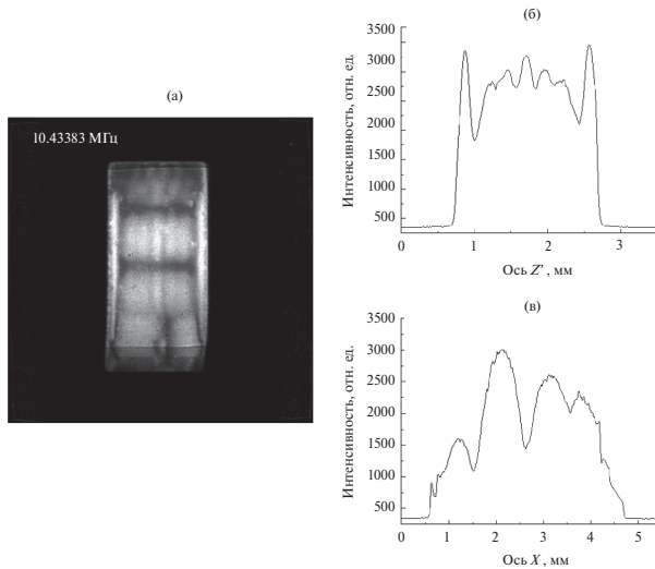
Рис. 6. (а) — Топограмма и (б), (в) — графики распределения по двум направлениям амплитуды деформаций пьезоэлемента на резонансной частоте 10.43383 МГц, соответствующей ангармоническому колебанию.
