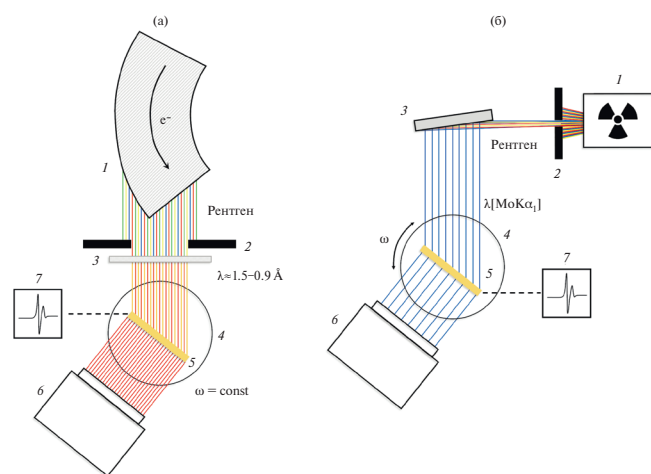
Рис. 2. Схемы реализации измерений. (а) — Топография на белом пучке в однокристалльной схеме дифракции, реализованная на синхротронной станции «Медиана» КИСИ-Курчатов. 1 — поворотный магнит, 2 — входная маска белого пучка, 3 — алюминиевый фильтр для поглощения длинноволновой части спектра, 4 — гониометрическая система, 5 — образец с держателем, 6 — двумерный детектор, 7 — генератор/анализатор электрического сигнала. (б) — Топография на монохроматическом пучке в двухкристалльной схеме дифракции, реализованная на лабораторном трехкристалльном рентгеновском спектрометре ТРС-К: 1 — рентгеновская трубка, 2 — щель предварительной коллимации, 3 — асимметричный однокристалльный монокроматор, 4 — гониометрическая система, 5 — образец с держателем, 6 — двумерный детектор, 7 — генератор/анализатор электрического сигнала.
