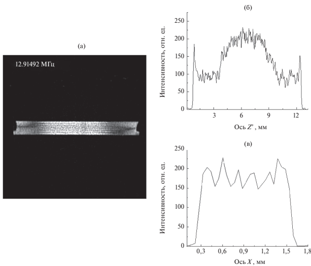
Рис. 9. (а) — Топограмма и (б), (в) — графики распределения по двум направлениям деформаций пьезоэлемента на резонансной частоте 12.91492 МГц.
