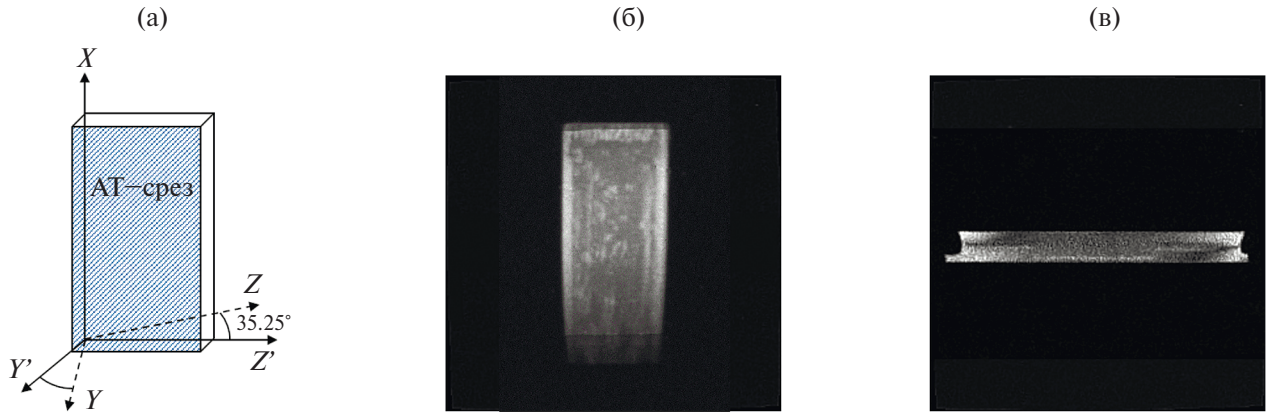
Рис. 3. (а) — Схематическое представление кристаллографической ориентации АТ-среза кварца; (б) и (в) — исходные топограммы резонаторов РК563 и РК319 соответственно, полученные в нормальных условиях (без внешнего воздействия).
